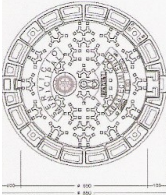
INSTALACIÓN EN CALZADA Clase D400
